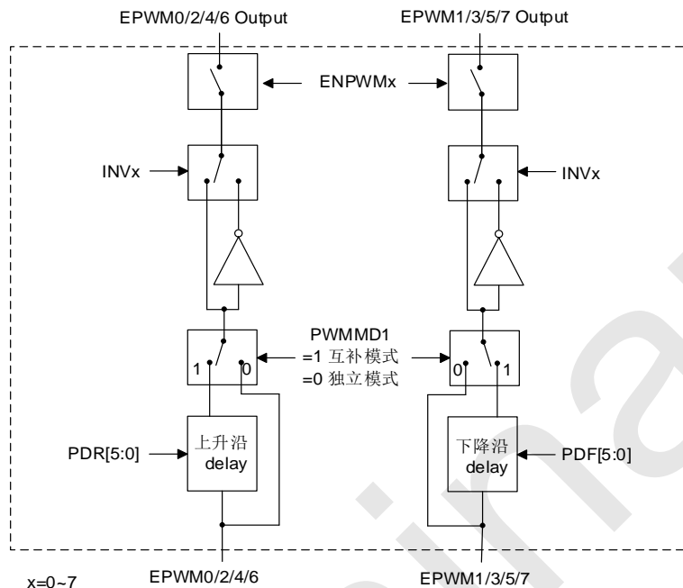
SCD515X 系列 EPWM 互补模式框图
