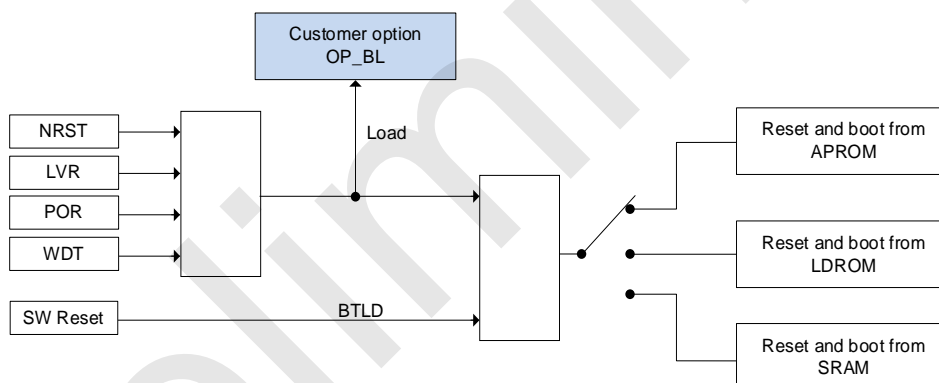
SCD515X 复位后启动区域切换示意图
