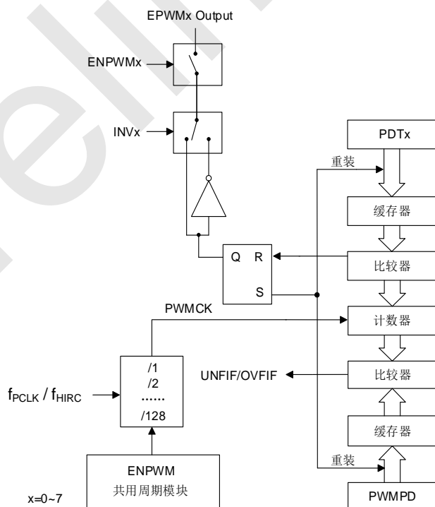
SCD515X 系列 EPWM 独立模式框图
