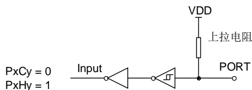
带上拉的输入模式
